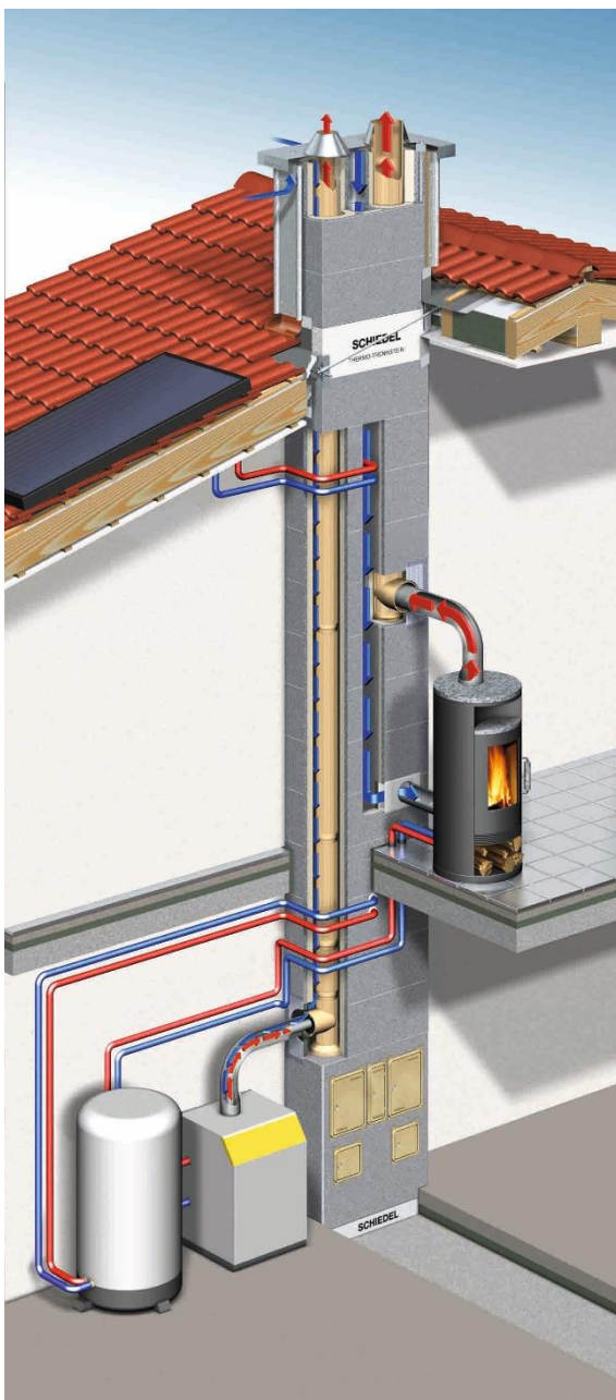
Ein Schornstein erhöht die Flexibilität und Unabhängigkeit bei der Wärmeversorgung
